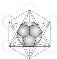
Fig. 6-21a. Solid dodecahedron.
